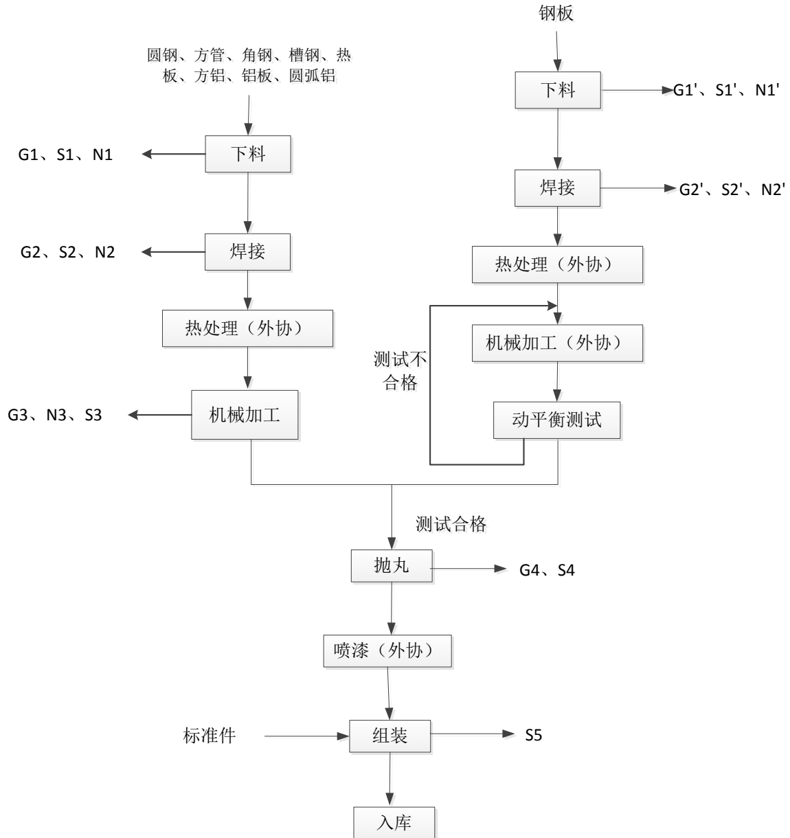
图 5-1 生产工艺流程及产污环节图
