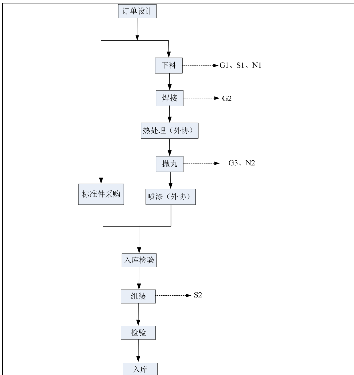
图 1-2 生产工艺流程及产污环节图
