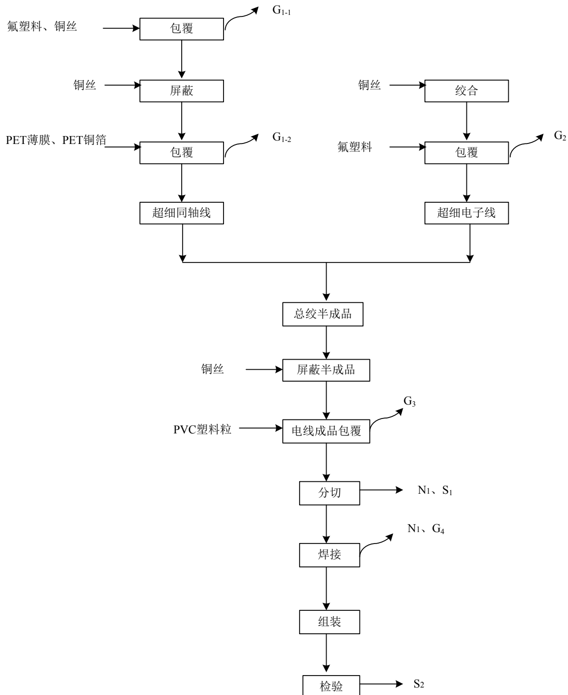
图 5-1 项目工艺流程图
