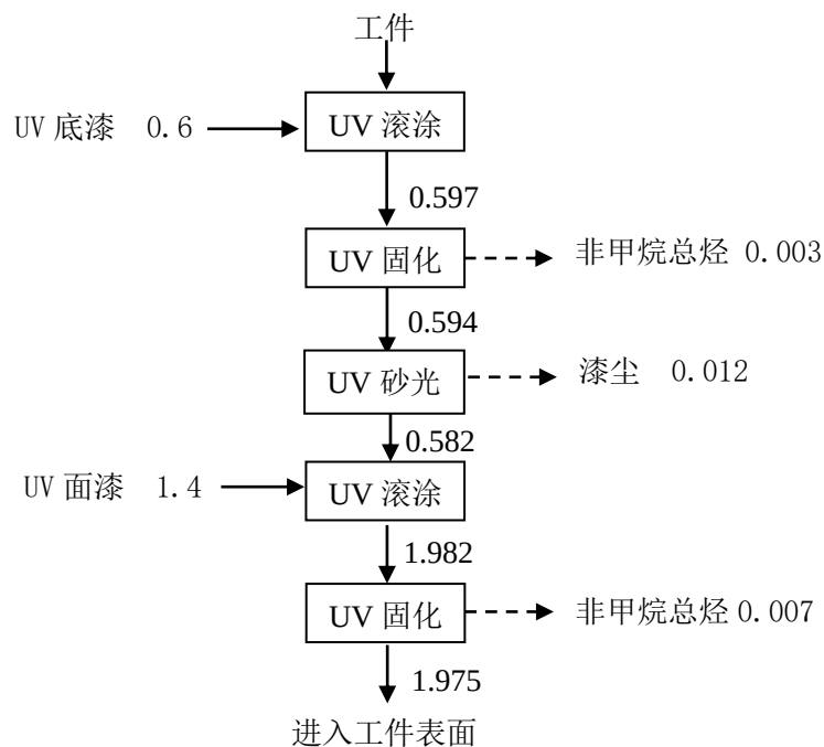
图 5-2 UV 漆物料平衡图 (t/a)
