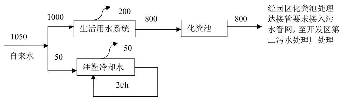
图 5-2 项目用水及排水平衡图（单位：t/a）
