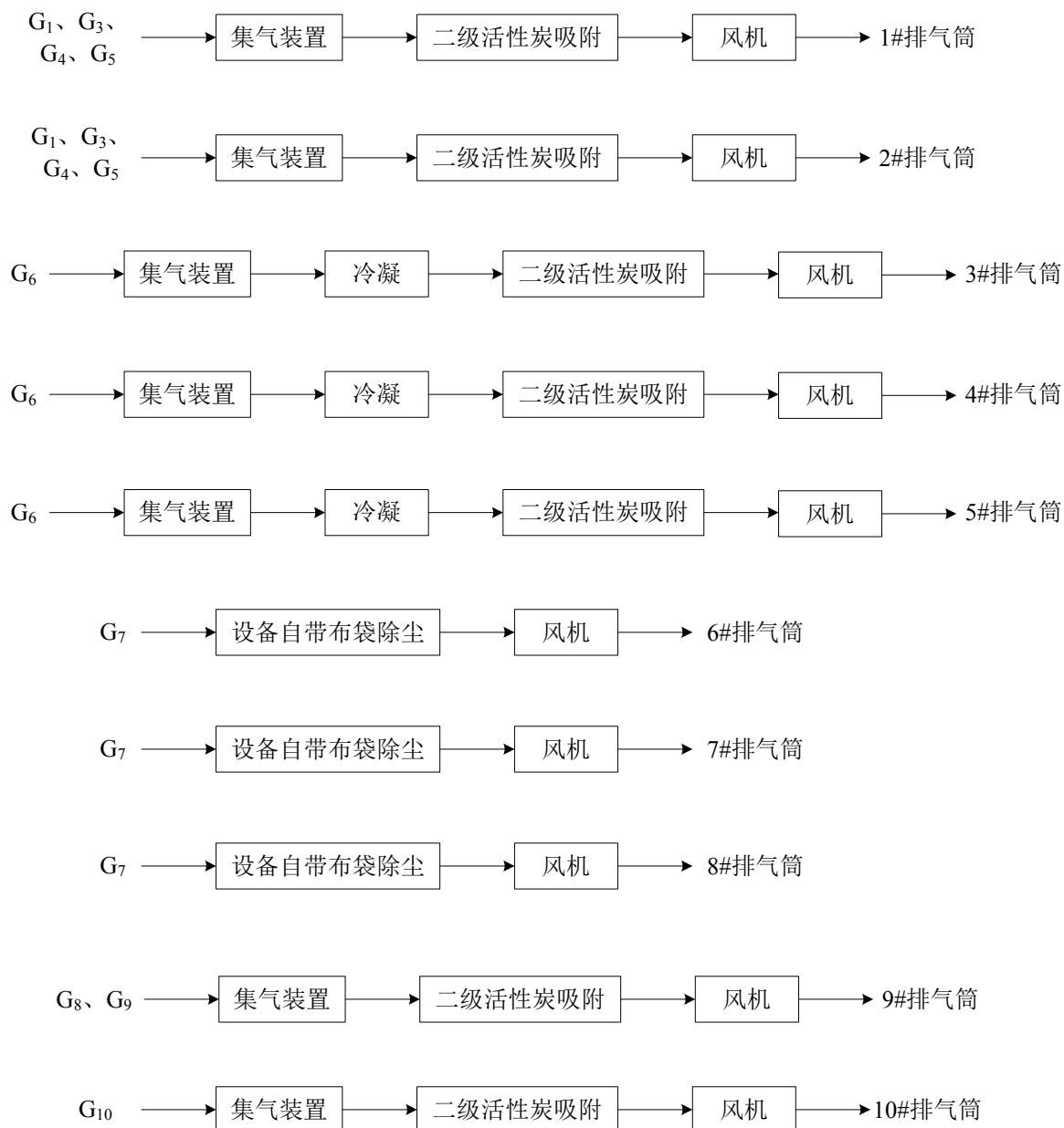
图8.1-1 本项目废气收集、处理和排放系统示意图
