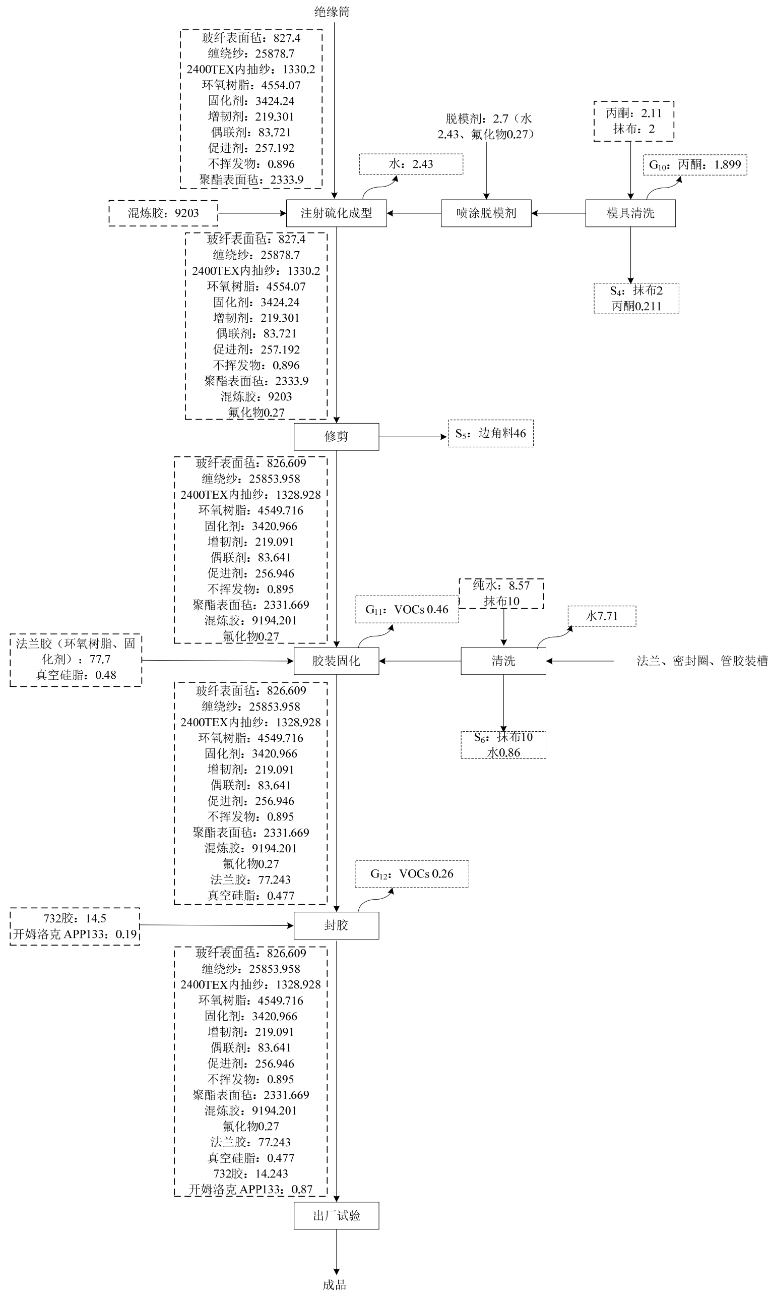
图 4.3-2 成型工艺物料平衡 (t/a)
