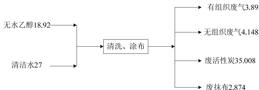
图 4.3-3 乙醇平衡图 (t/a)
