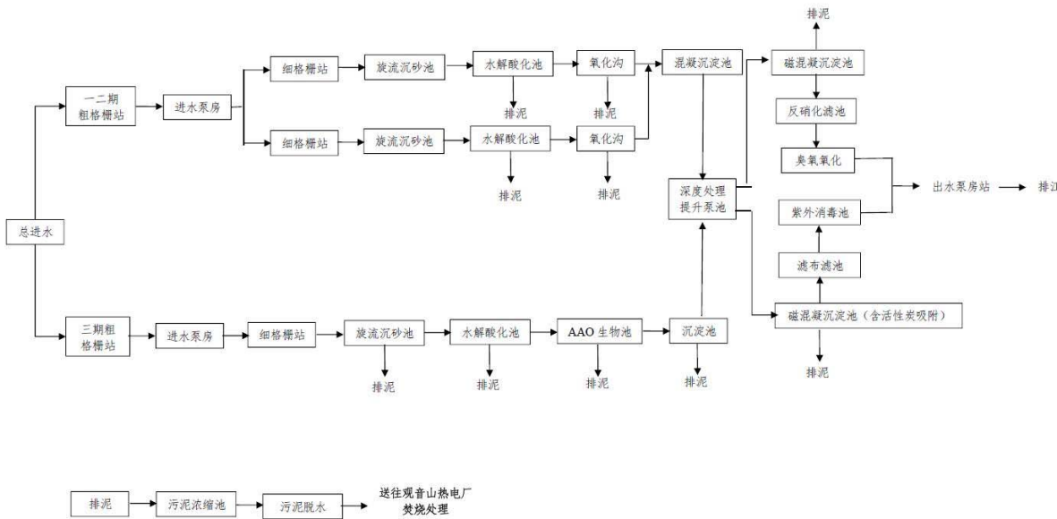
图 8.2-1 开发区第二污水处理厂污水处理工艺流程图
